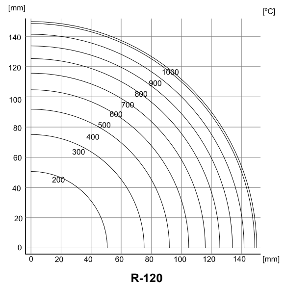
Figura C.7. Isotermas de un cuarto de sección circular de 300 mm de diámetro expuesta perimetralmente
