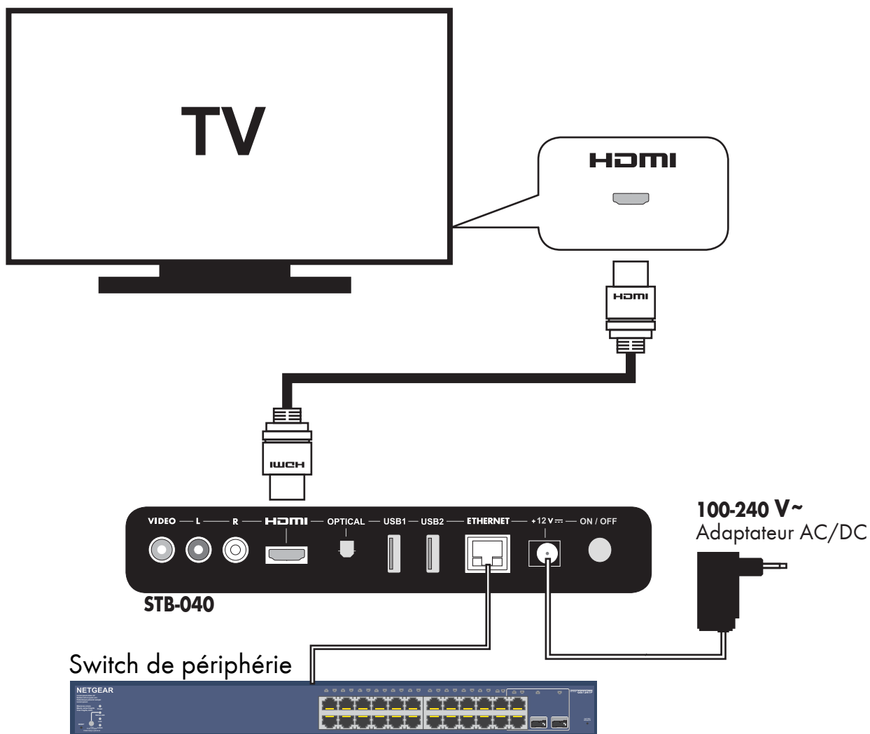
Fig. 2 – Connexion HDMI
