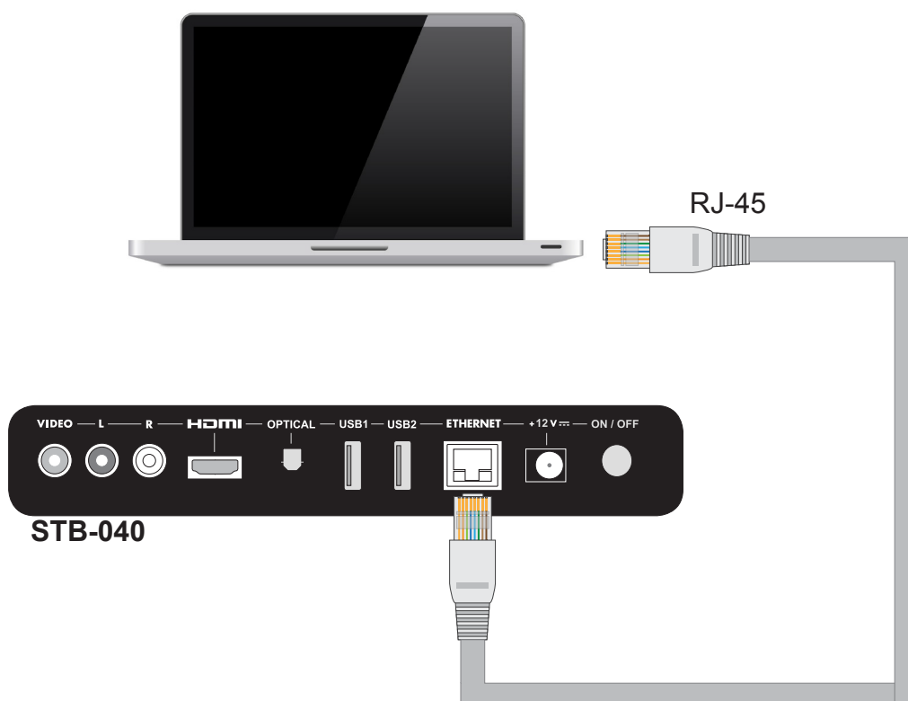
Fig. 10 - Conexión directa entre PC y STB-040
