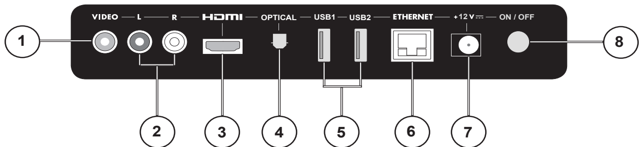
Fig. 1 – Verso STB-040
